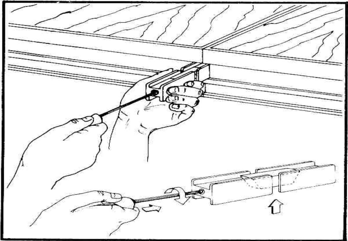
Bild 1: Anwendung der Klemmfix-Podestverbinder
