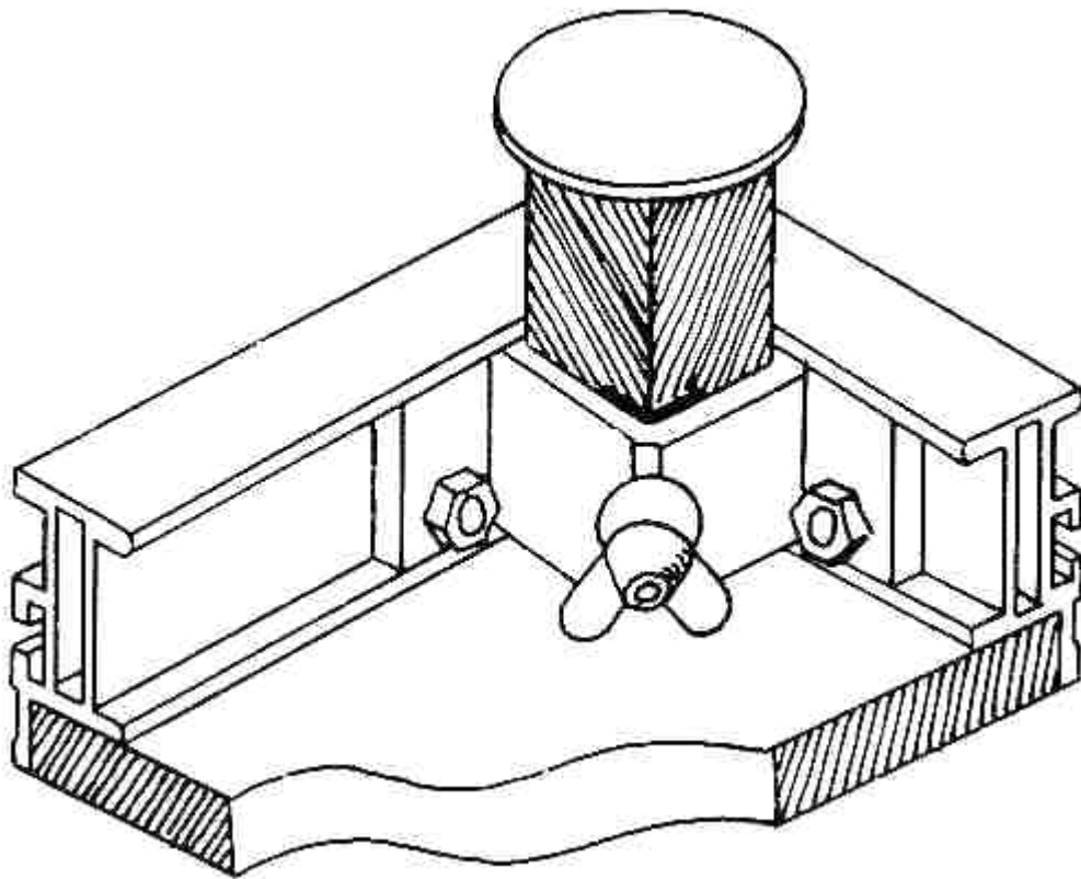
Bild 3: Druckgussecke zur Aufnahme der Steckfüße
