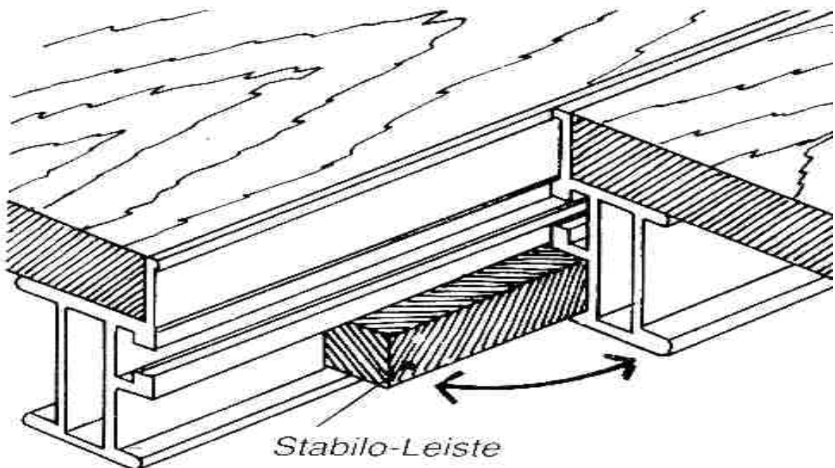
Bild 2: Anwendung der Stabilo-Leisten
